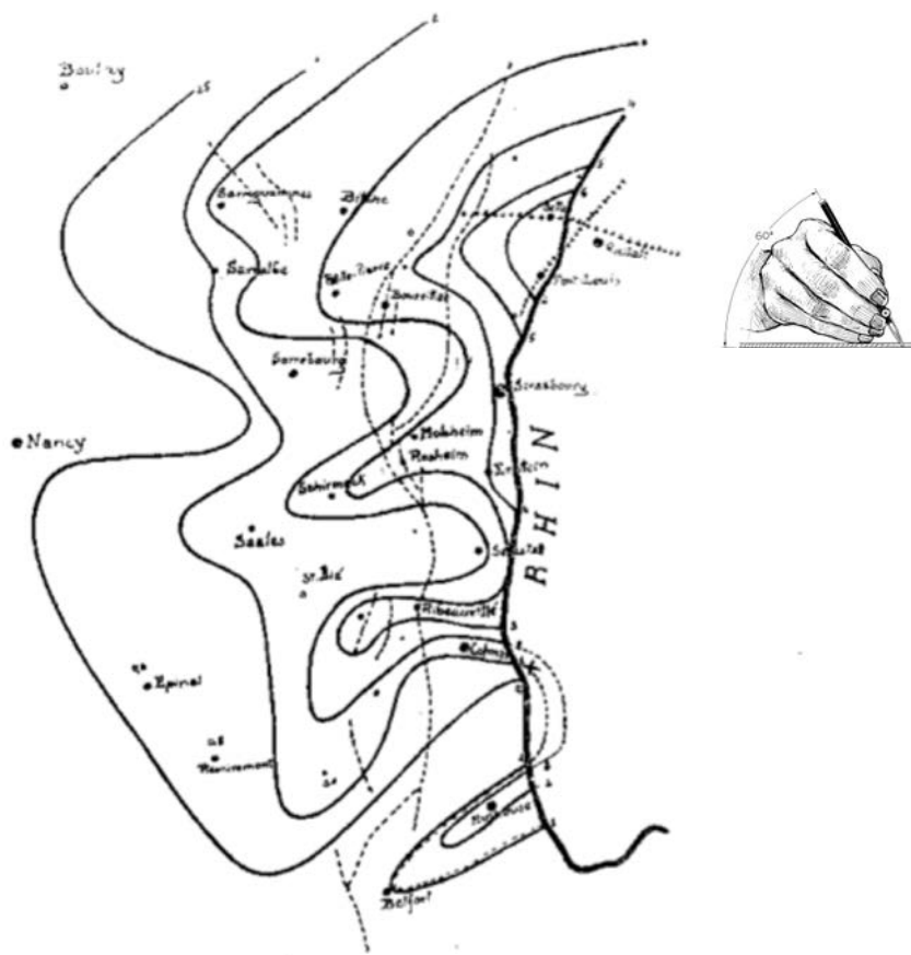
Fig. 1. Lignes isoséistes
